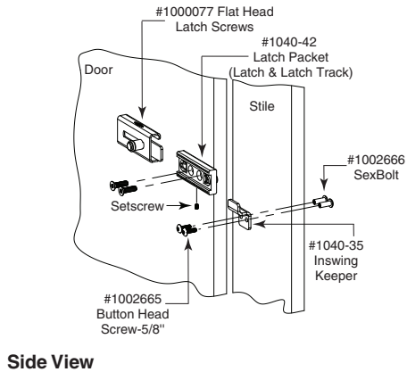
Fig. 10e: INSWING Door Keeper for Inline Stiles.
