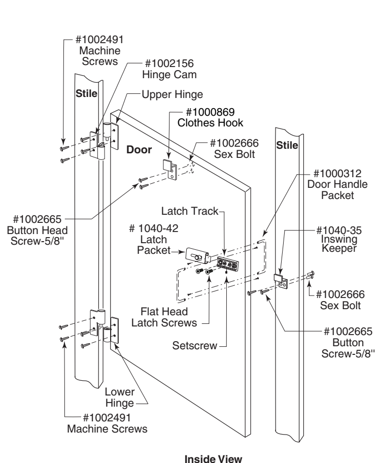
Fig. 10a: INSWING Door Hardware. (example)
